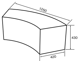
スネーク SL-5SN 14,200 W1250×D420×H430mm RGBW LED 消費電力：10W
