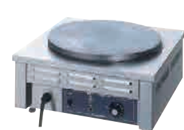
電気クレープ焼器 US-39CS 48,000 W500×D500×H200mm 質量：31kg 消費電力：1.4kw 電源：単相100V
