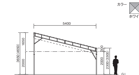
片屋根テント(3x4K) OS-06KE 面積：38.88㎡
