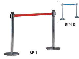
ベルトリールパーティション 4,400 BP-1 (レッド) BP-1B (ブルー) φ300×H877mm 1本 ベルト2m
