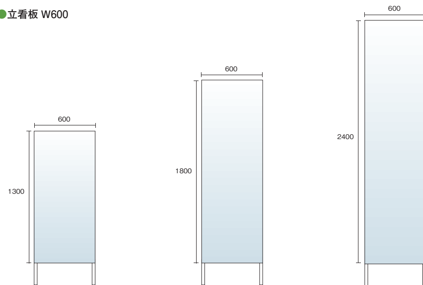
立看板 H1300
