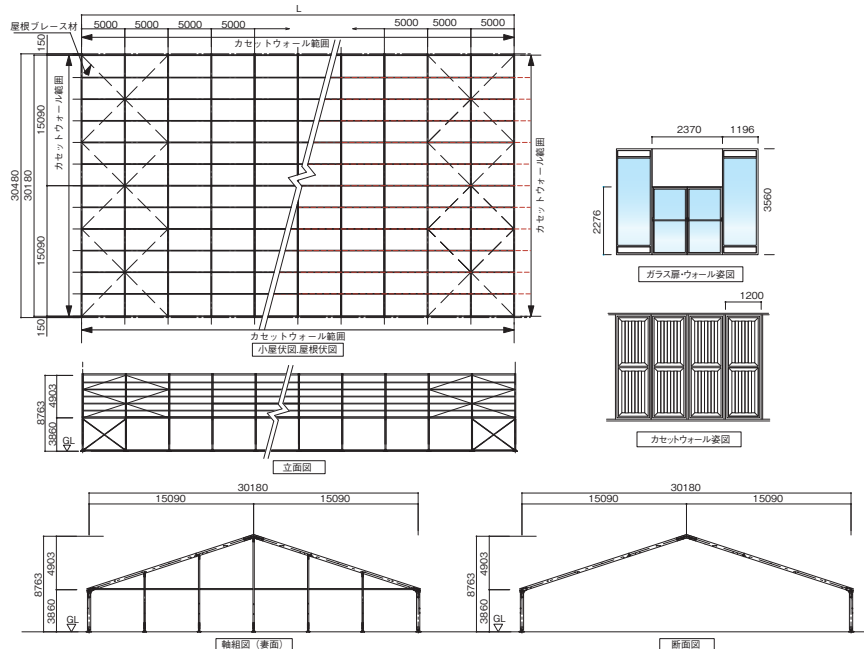
マキシフレックス(30m) OS-02OM
