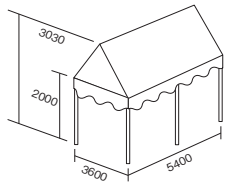
パイプテント(2×3K) OS-11KE
