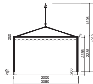
軸組図
