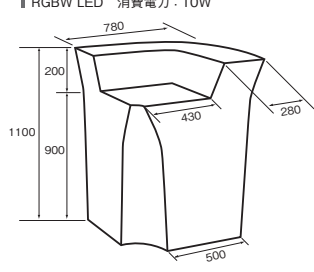
コーナーBAR SL-4COB 38,400
