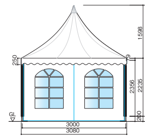
立面図 (横幕付)
