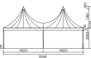
立面図
