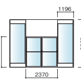
ガラス扉・ウォール姿図
