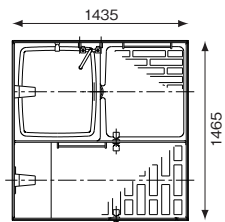
ユニットバス OS-04TU 重量：104kg
