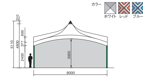
テント(8m) OS-04KE 面積：64㎡
