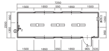
単体ハウス(5.1坪) OS-05NG W7250×D2300×H2603mm 質量: 1400kg 床荷重: 298kg/m 2
