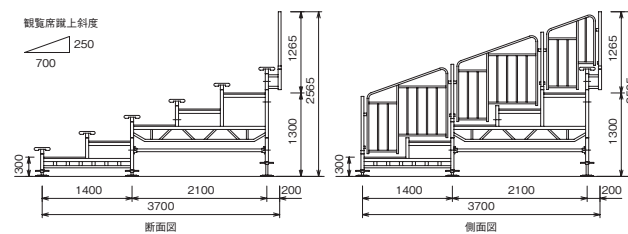
仮設スタンド OS-01AL
