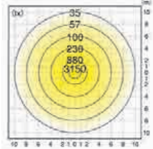
照明測定分布図
