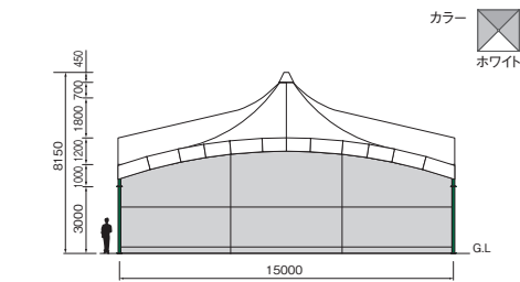
ビッグパワーテント(15m) OS-02KE 面積：225㎡
