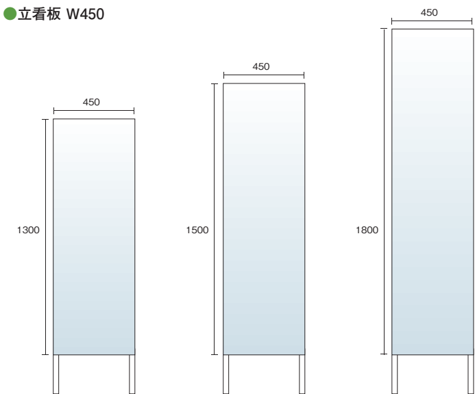
立看板 H1300
