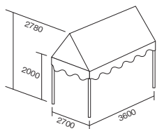
パイプテント(1.5×2K) OS-12KE
