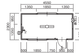
単体ハウス(3.2坪) OS-03NG W4550×D2300×H2603mm 質量: 1000kg 床荷重: 298kg/m 2
