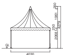
立面図
