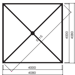
平面図 (床伏せ図)
