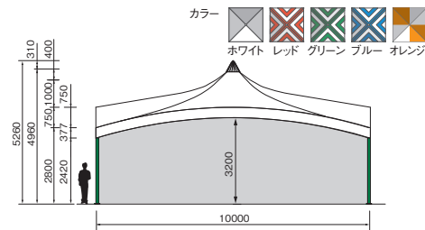
ビッグパワーテント(10m) OS-03KE 面積：100㎡
