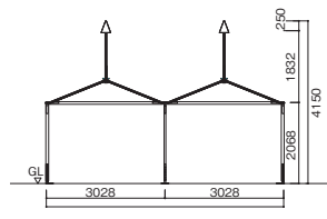
軸組図
