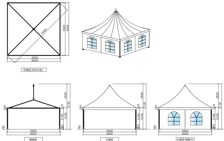
ヨーロッパン・シャレー(6m) OS-05OM
