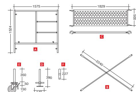
イントレ OS-01WD
