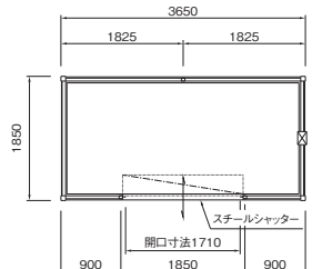
物置ハウス(2.0坪) OS-07NG W3650×D1850×H2603mm 質量: 680kg 床荷重: 616kg/m 2
