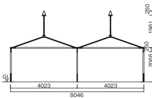
軸組図
