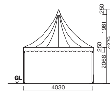
立面図
