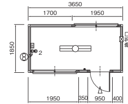
単体ハウス(2.0坪) OS-02NG W3650×D1850×H2603mm 質量: 720kg 床荷重: 616kg/m 2
