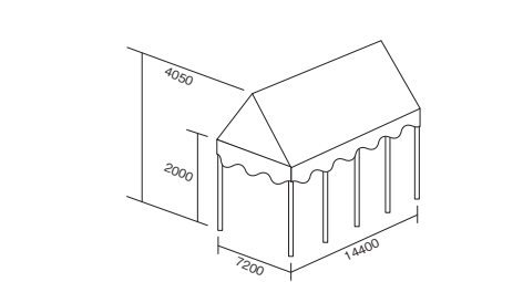
パイプテント(4Kx8K) OS-07KE 面積：103.7㎡
