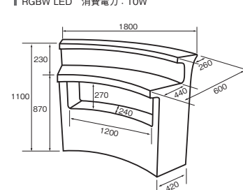
ブレイクBAR SL-4BRB 38,500
