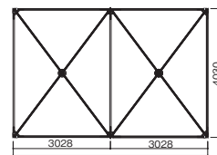
平面図 (床伏せ図)
