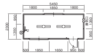
単体ハウス(3.8坪) OS-04NG W5450×D2300×H2603mm 質量: 1110kg 床荷重: 298kg/m 2
