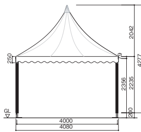
立面図
