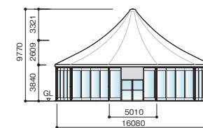
立面図
