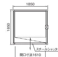
物置ハウス(1.0坪) OS-06NG W1850×D1850×H2603mm 質量: 450kg 床荷重: 616kg/m 2
