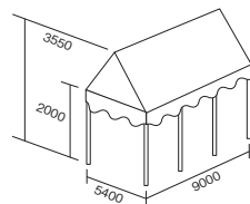
パイプテント(3×5K) OS-09KE
