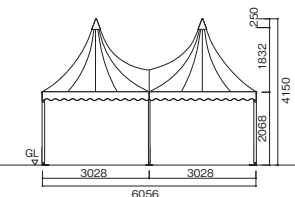
立面図
