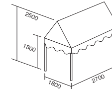
パイプテント(1×1.5K) OS-13KE
