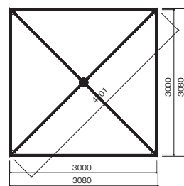
平面図 (床伏せ図)
