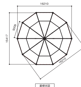
屋根伏図
