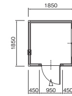
単体ハウス(1.0坪) OS-01NG W1850×D1850×H2603mm 質量: 460kg 床荷重: 616kg/m 2
