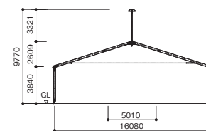
断面図
