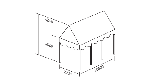
パイプテント(4Kx6K) OS-08KE 面積：77.8㎡
