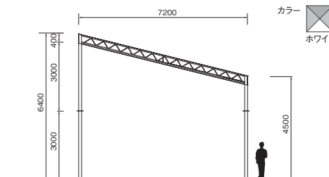
片屋根テント(10x7.2m) OS-05KE 面積：72㎡
