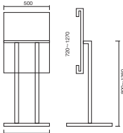
パネルスタンド SS-3 5,200 W500×D430×H800~1350mm パネル: W500~900×H720~1270mm 厚さ30mm
