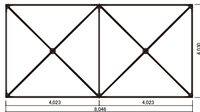
平面図(床伏せ図)
