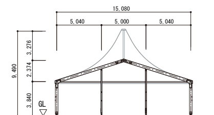
軸組図 (妻面)
