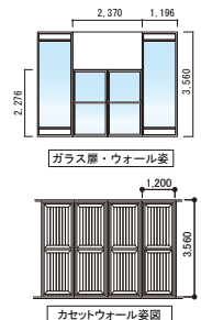
カセットウォール図
