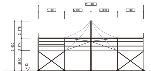
立面図
