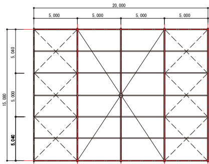
小屋伏図, 屋根伏図
