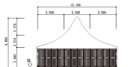
立面図 (妻面)
